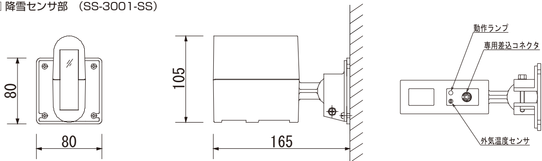
□ 降雪センサ部 (SS-3001-SS)
