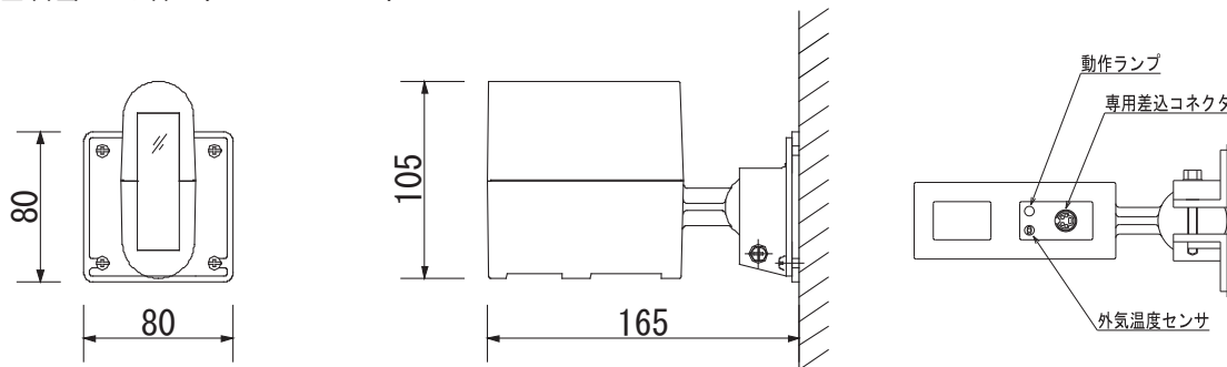
□ 降雪センサ部（SS-3001-HTS）
