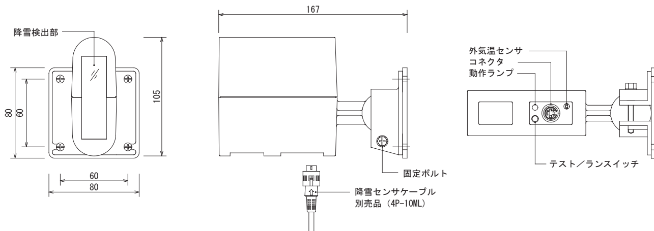
□ 降雪センサ部 (SS-3200-SS)
